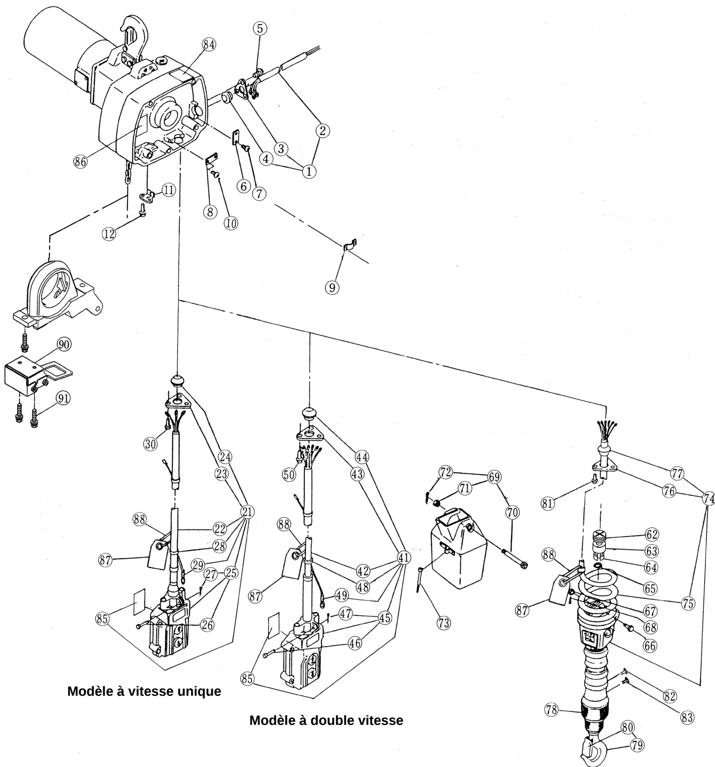
Modèle à cylindre double vitesse
